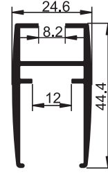
7005 E 0.610 kg/m Tek Camlı Sürgü Profili
