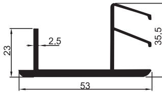
7022 A 0.660 kg/m Amortisörlü Arka Sürgü Kanalı
