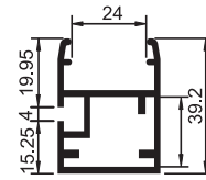
8019 Sürgü Kanalı Renk Seçeneği: Gri veya Siyah
