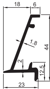
7016 0.410 kg/m Raf Tırnağı
