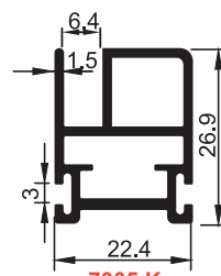
7005 K 0.440 kg/m Tek Cam Kanat Profili
