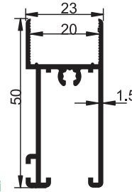
7005 L 0.632 kg/m Isıcamlı Sürgü Profili
