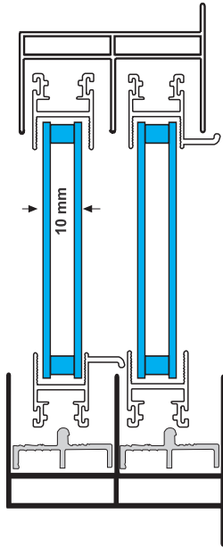
7005 F 0.410 kg/m Isıcam Kanat Profili
