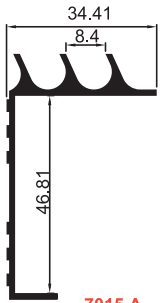
7015 A 0.610 kg/m Sürgü Kanalı
