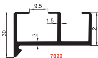
7022 0.670 kg/m Sürgü Kanalı
