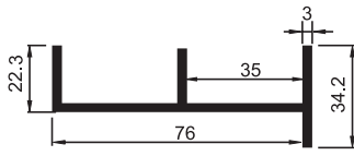
8017 Alt Ve Üst Ray Renk Seçeneği: Gri veya Siyah
