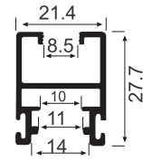
9007 D 0.378 kg/m Tek Cam Kanat Profili
