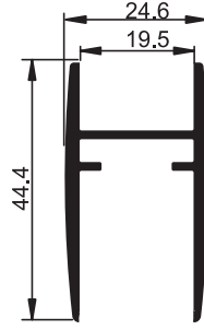
7005 0.820 kg/m Isıcamlı Sürgü Profili
