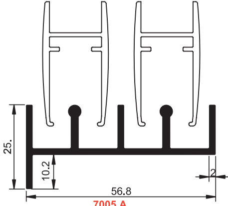
7005 A 0.820 kg/m Tek Camlı Sürgü Profili
