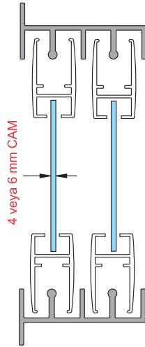
7005 L 0.632 kg/m Isıcamlı Sürgü Profili
