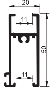
7005 C 0.660 kg/m Isıcamlı Sürgü Profili
