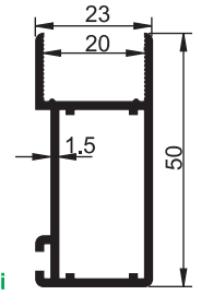
7005 M 0.629 kg/m Isıcamlı Sürgü Profili
