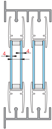
7005 D 0.653 kg/m Tek camlı Sürgü Profili
