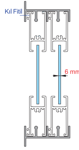
7005 M 0.629 kg/m Isıcamlı Sürgü Profili
