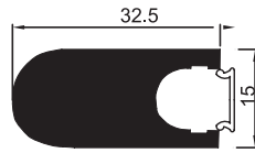
7020 1.170 kg/m Kablo Kanallı Önden Destek Laması
