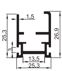
7005 F 0.410 kg/m Isıcam Kanat Profili
