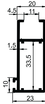
7005 D 0.653 kg/m Tek camlı Sürgü Profili
