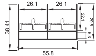
7005 G 0.660 kg/m Üst Ray
